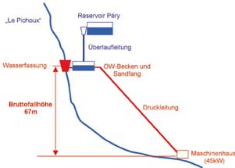
Bild 4: Nutzung eines Reservoirüberlaufes mit zusätzlicher Bachfassung
