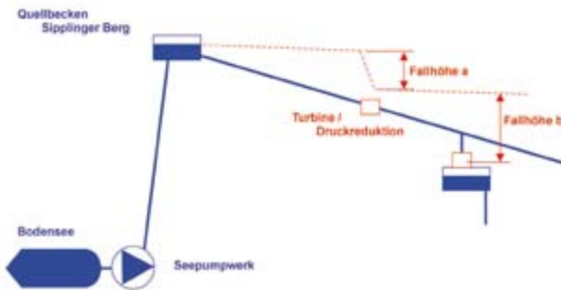
Bild 5: Prinzip der Wasserkraftnutzung in Pumpsystemen am Beispiel der Bodensee-Wasserversorgung mit a) Turbine in Hauptleitung und b) Turbine in Reservoir einlauf (Nutzung der Restenergie)
