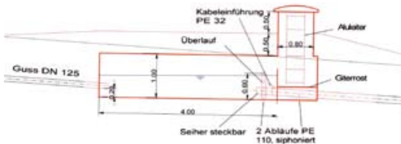
Bild 9: Schnitt durch ein neu erstelltes Oberwasserbecken für ein Trinkwasserkraftwerk.
