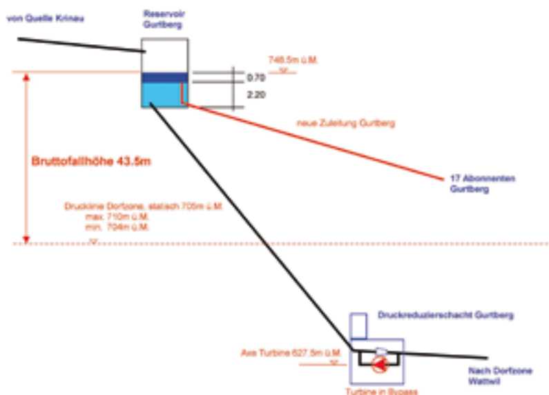
Bild 3: Wasserzufluss von einem hoch liegenden Reservoir direkt in das Dorfnetz. Einsatz einer Turbine parallel zum Druckreduzierventil, welches unter dem Gegendruck des Dorfnetzes arbeitet; auch die Turbine muss unter dieser Bedingung funktionieren können.
