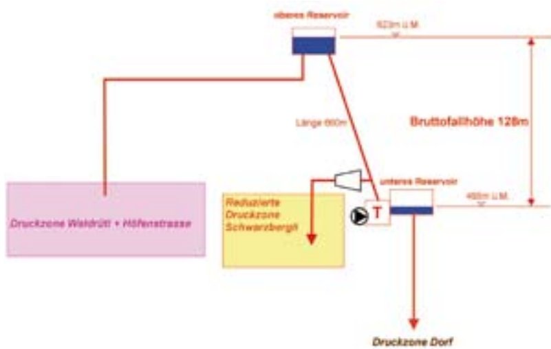
BILD 2: Wassertransfer zwischen zwei Reservoiren einer Wasserversorgung. Einsatz einer Turbine (T) parallel zum geregelten Druckhalteventil, welches das Entleeren des oberen Reservoirs verhindert.
