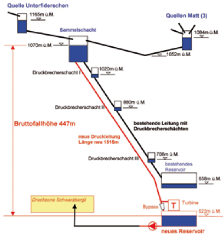
Bild 1: Typische Situation einer Wasserversorgung mit hoch liegenden Quellen, die ein Dorf im Tal versorgen. Die ursprünglich in Druckbrecherschächten vernichtete Energie kann mittels einer Turbine (T) in Strom umgewandelt werden. Das Kraftwerksprojekt wird erst im Zuge der Erneuerung der Druckleitung und des Reservoirs umgesetzt.
